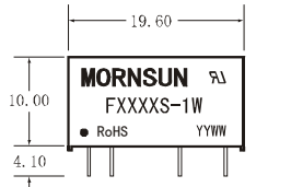
FXXXXS-1W 封装
