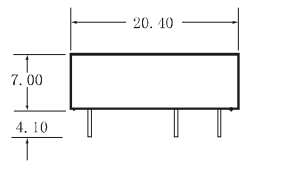
FXXXXD-1W 封装
